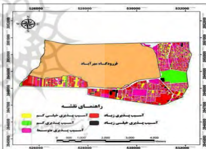
نگاره ۶: آسیب وارده در زلزله‌ی با ۷ مرکالی
