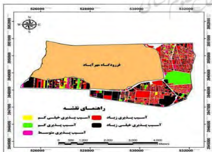
نگاره ۶: آسیب وارده در زلزله‌ی با ۷ مرکالی
